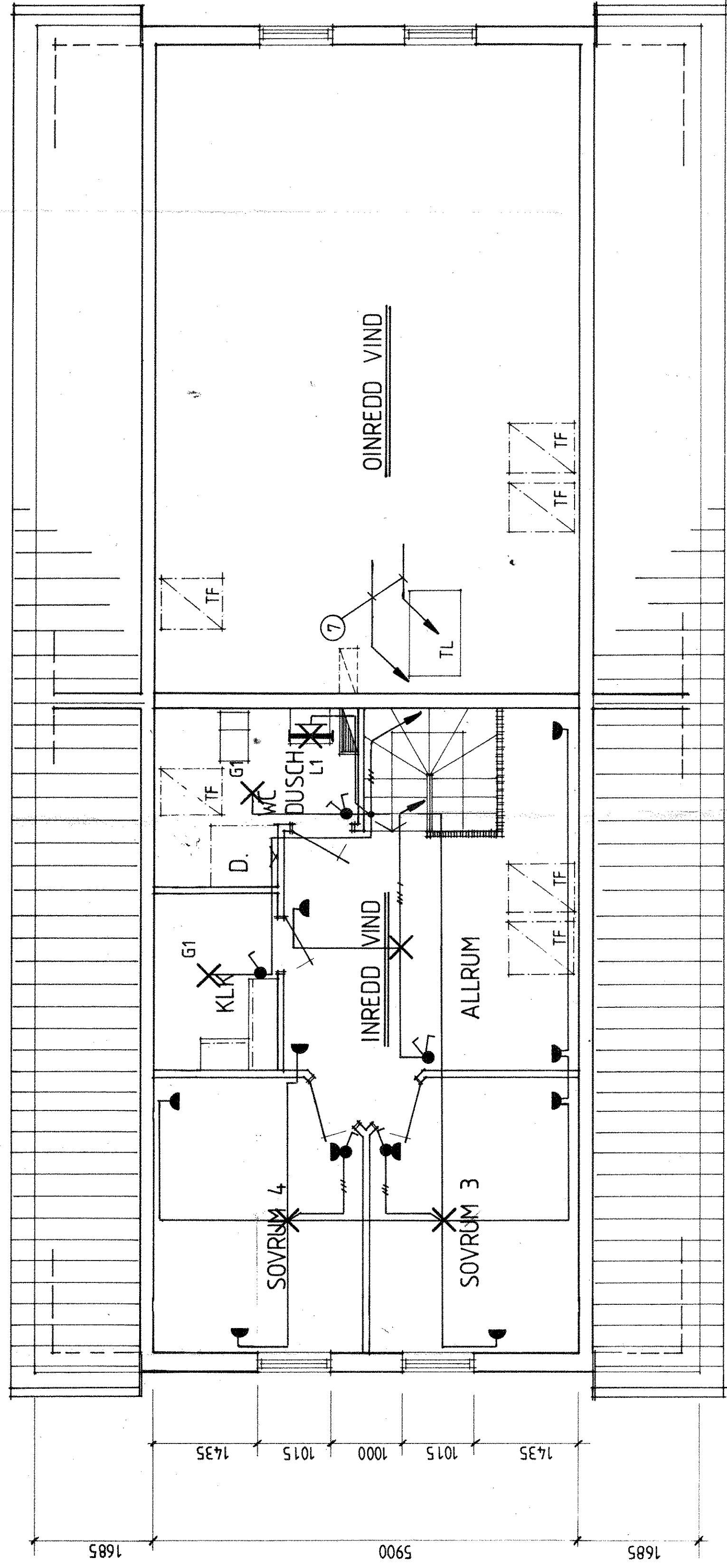
HUS A VINDSVÅNING 1:50
